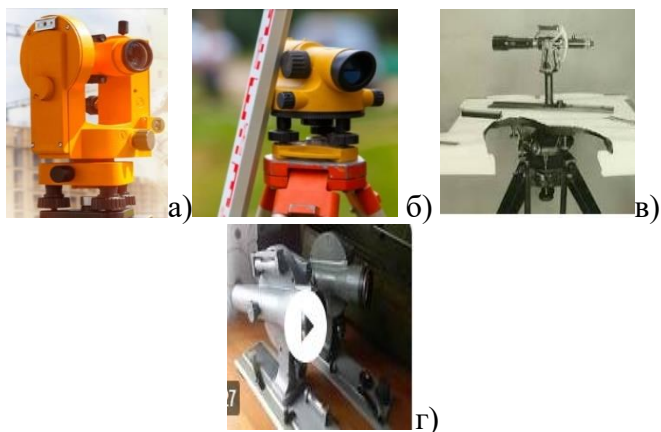
Рис.3. Механічні геодезичні прилади а) – теодоліт; б) – нівелір; в) – мензула; в) кіпрегель
