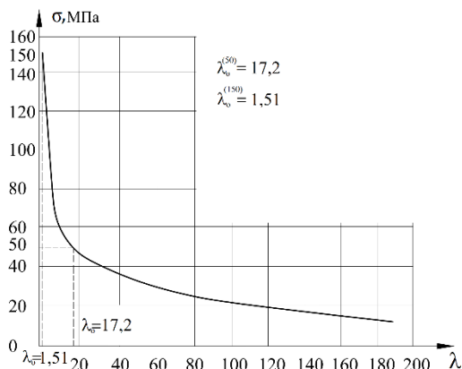
Рис. 1. Графік залежності руйнування напружень \sigma від гнучкості \lambda бетонних колон у склопластиковій обоймі
