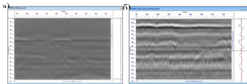
Рис. 1. Візуалізація радарограми у програмі «GPR Proview»: а) до первинної обробки; б) після первинної обробки
