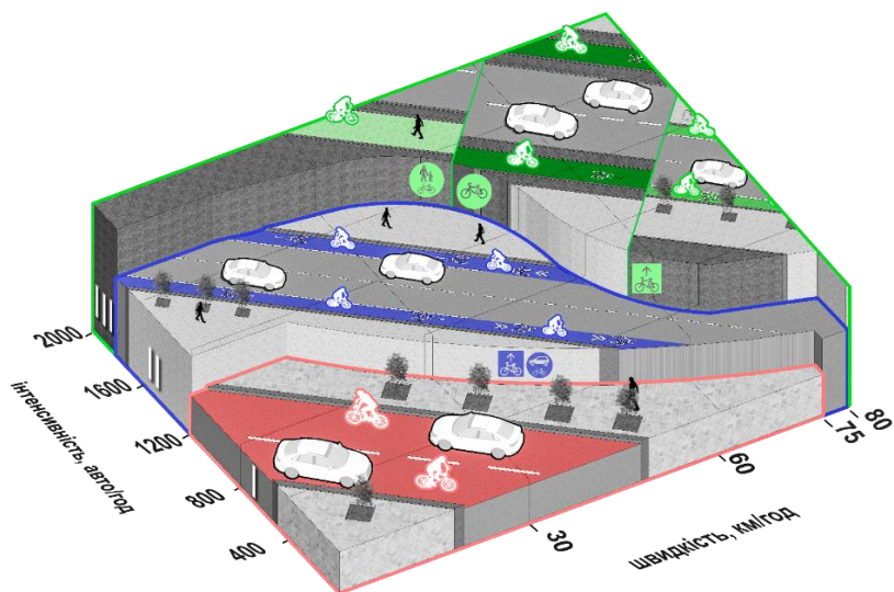
Рис. 1 Схема вибору форми велосипедного руху в залежності від швидкості та інтенсивності автомобільного транспорту на вулиці з двома смугами руху
